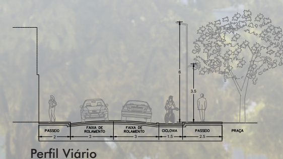
Perfil Viário
